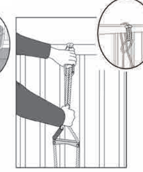
手摺にオリロープを巻いてカラビナを2本のロープに取り付ける。
