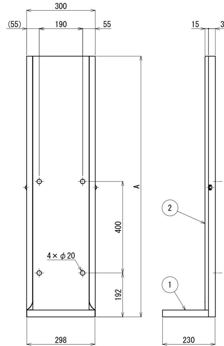
本体 (固定部)
