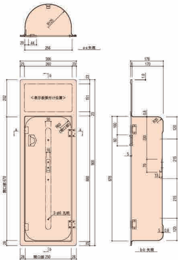
OB.1 寸法図
