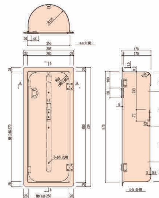
OB.2 寸法図
