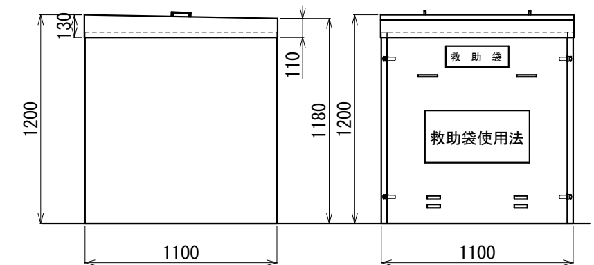
分解型格納箱寸法図 ボンデ鋼板 t 1.2 粉体塗装仕上
