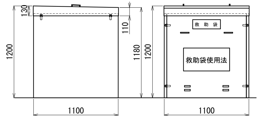
分解型格納箱寸法図
