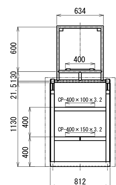
入口金具及び取付具 サビ止塗装及び吹付塗装仕上 上塗 ニューハイメル (N-30近似色 グレー) 下塗 1液ハイポンファインデクロ (赤錆)
