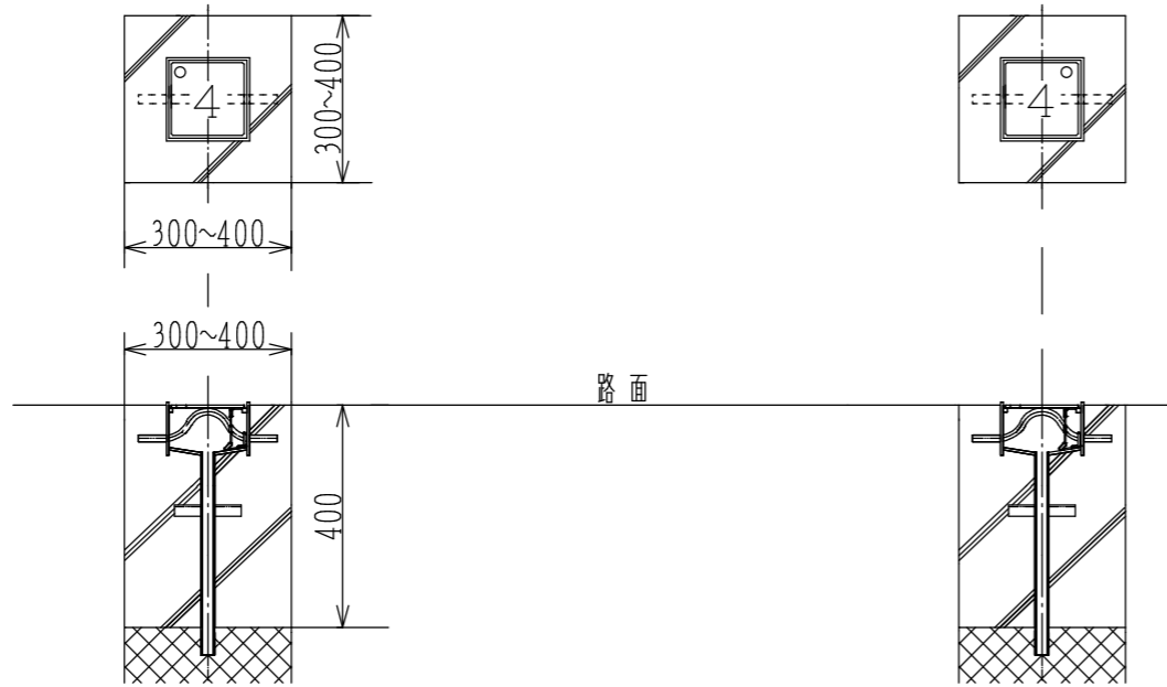
固定環埋設図 S: 1/10
