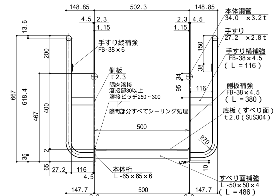
【B-B 断面】
