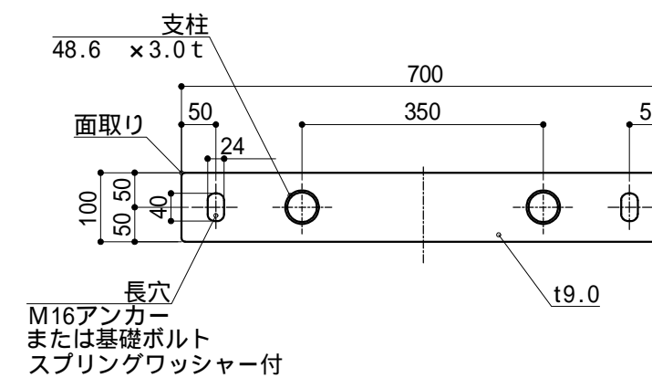
【ベース板 平面】
