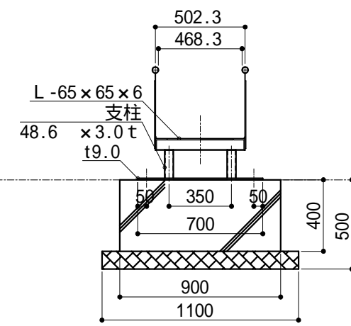
【出口部 断面】
