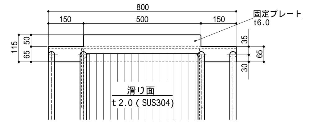
【乗込み部 平面】
