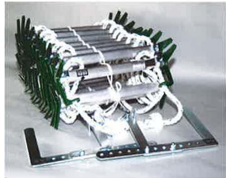
オリールII型
