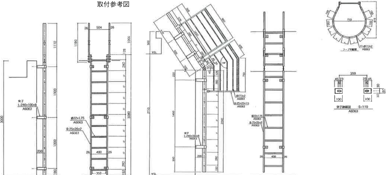
アルフィクス
