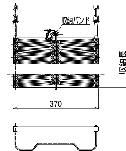
収納姿図
